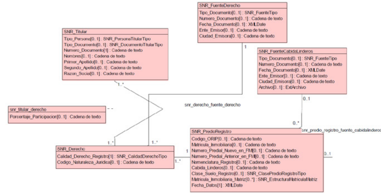
Figura 54. Submodelo de información insumo del SNR en el MALC versión 1.0. Fuente: ICDE (2024).
