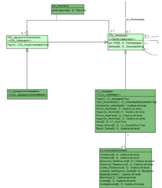
Figura 45. Paquete de interesados en el MALC versión 1.0. Fuente: a partir de IGAC (2024a).
