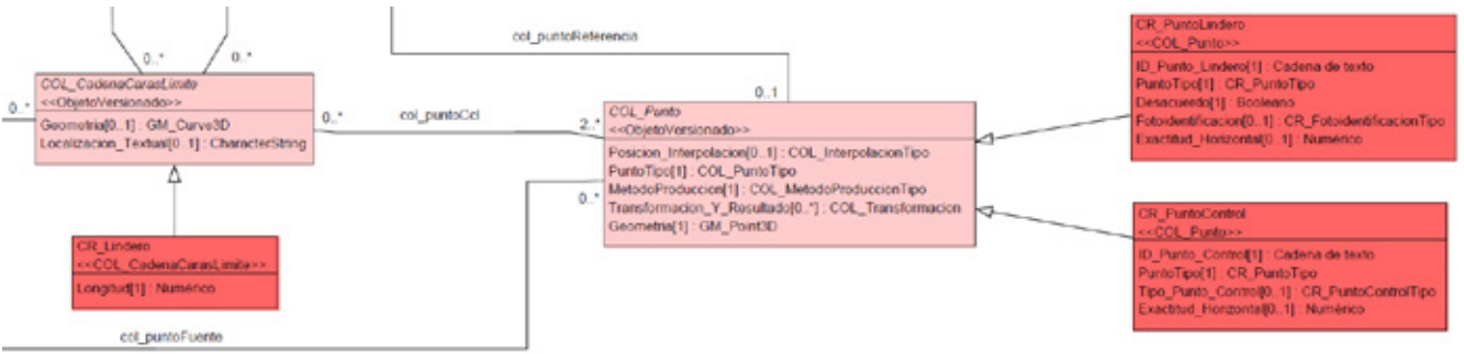
Figura 69. Subpaquete de topografía y representación MECR versión 4.0. Fuente: ICDE (2024).
