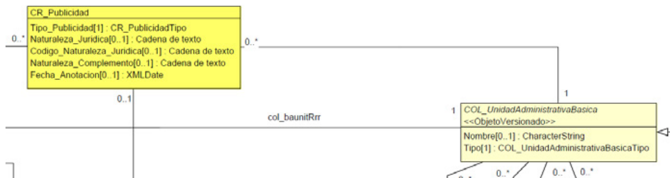
Figura 60. Clase “CR_Publicidad” del paquete administrativo MECR versión 4.0. Fuente: ICDE (2024).
