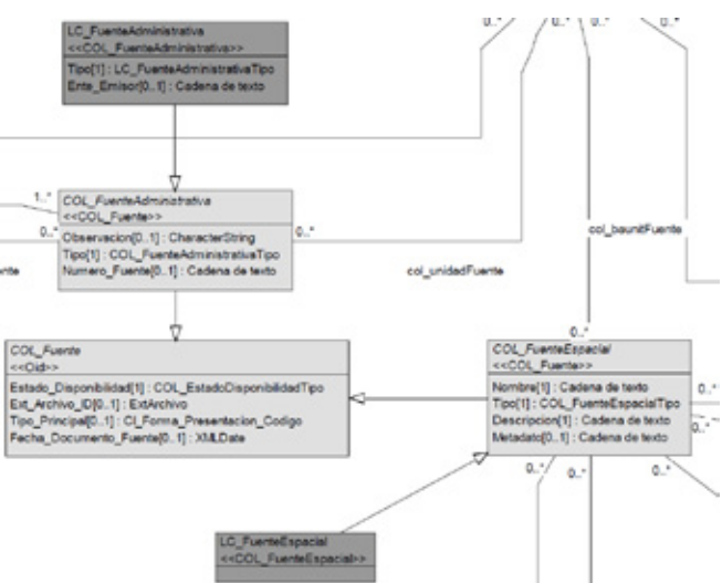
Figura 47. Componente de soporte documental del MALC versión 1.0. Fuente: a partir de IGAC (2024a).
