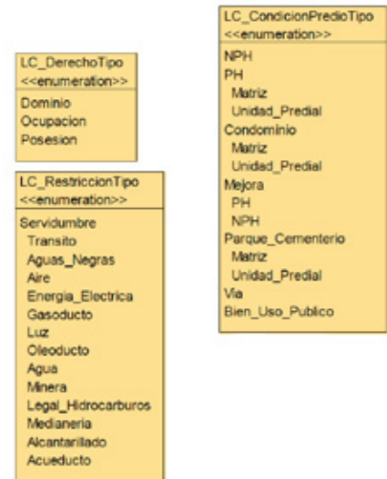
Figura 44. Dominios del paquete administrativo en el MALC versión 1.0. Fuente: IGAC (2024a).
