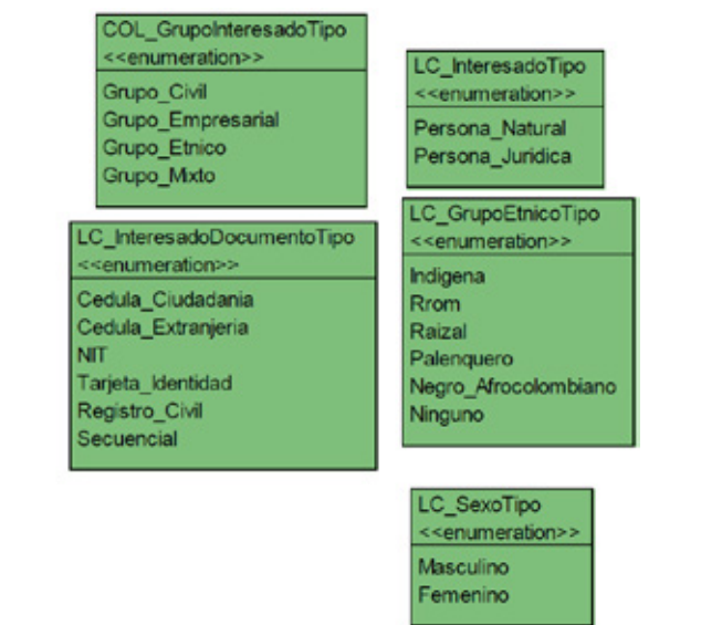
Figura 46. Dominios del paquete interesado del MALC versión 1.0. Fuente: a partir de IGAC (2024a).
